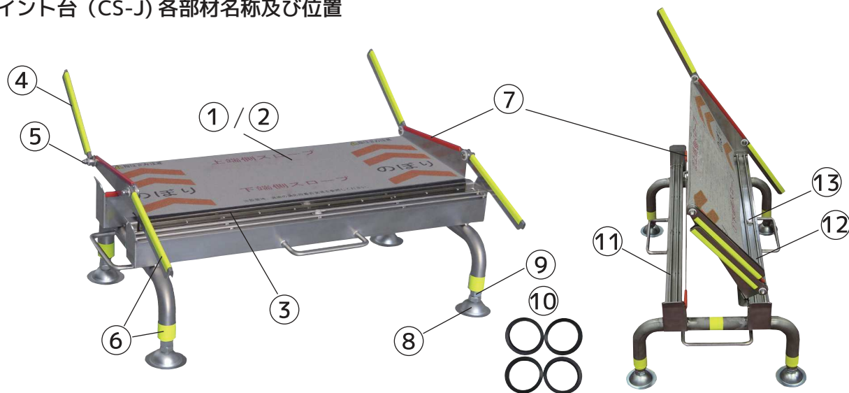
ジョイント台 (CS-J) 各部材名称及び位置
